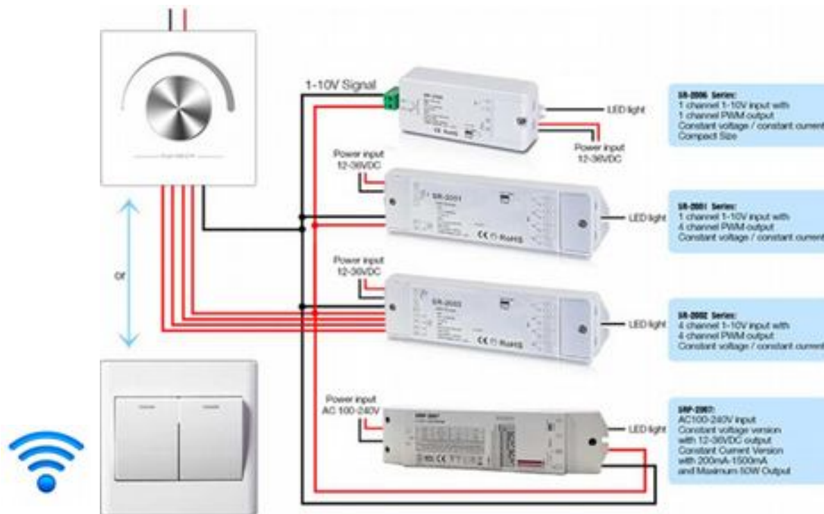
příklad zapojení stmívání s řízením 1-10V
